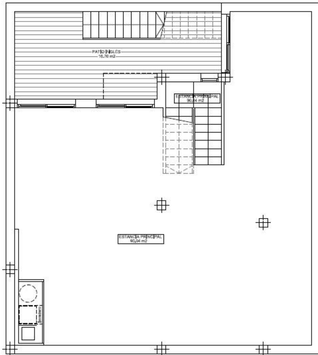
PLANTA SÓTANO
