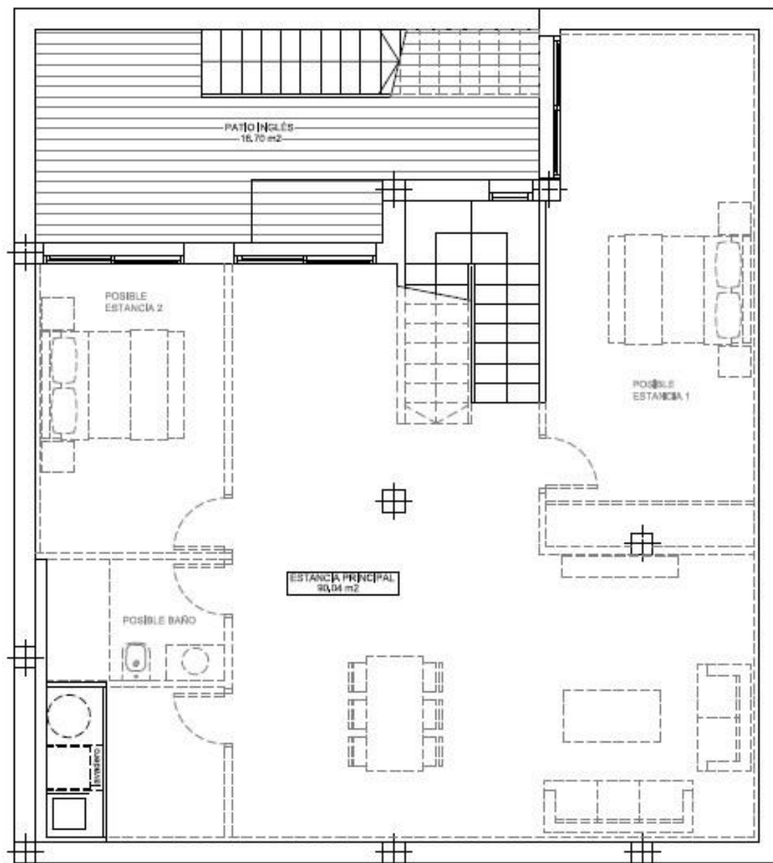
PLANTA SÓTANO, VIVIENDAS 19 Y 21 POSIBLE DISTRIBUCIÓN
